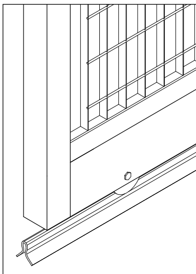
Guida sporgente dal pavimento
